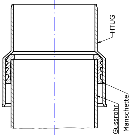
Einbausituation Teil 2
